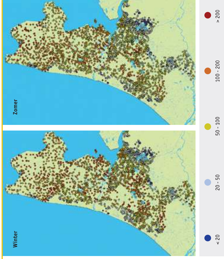
Figuur 5 gemiddelde sulfaatconcentratie in groeiseizoen en niet-groeiseizoen in \text{mg SO}_4 \text{ l}^{-1} . Gegevens van Rijnland, Krimpenerwaard, Waternet en Noordhollands Noorderkwartier.
