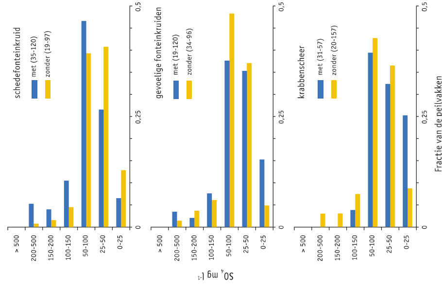
Figuur 4 frequentieverdelingen van het voorkomen van schedefonteinkruid ( Potamogeton pectinatus ), een groep gevoelige fonteinkruiden ( Potamogeton acutifolius , P. bercholdii , P. compressus , P. lucens , P. mucronatus en P. trichoides ) en krabbenscheer ( Stratiotes aloides ) bij verschillende klassen van sulfaatconcentraties gedurende het groeiseizoen in 207 peilvakken in de Noord-Hollandse Vechtstreek (gegevens WaterNet). Voor de peilvakken met en zonder planten wordt ook steeds de boven en onder 19%-percentiel sulfaatconcentratie gegeven. De frequentieverdelingen met en zonder waterplant zijn in alle drie de gevallen significant verschillend ( \chi^2 , P < 0.001 ).
