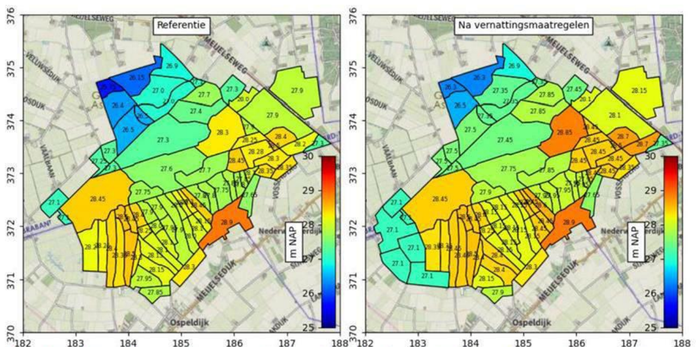
Figuur 3-13 Compartimentering in van de Groote Peel, met streefwaterpeilen voor en na nemen van vernattingsmaatregelen (Overgenomen uit: Stuurman et al., 2021)
