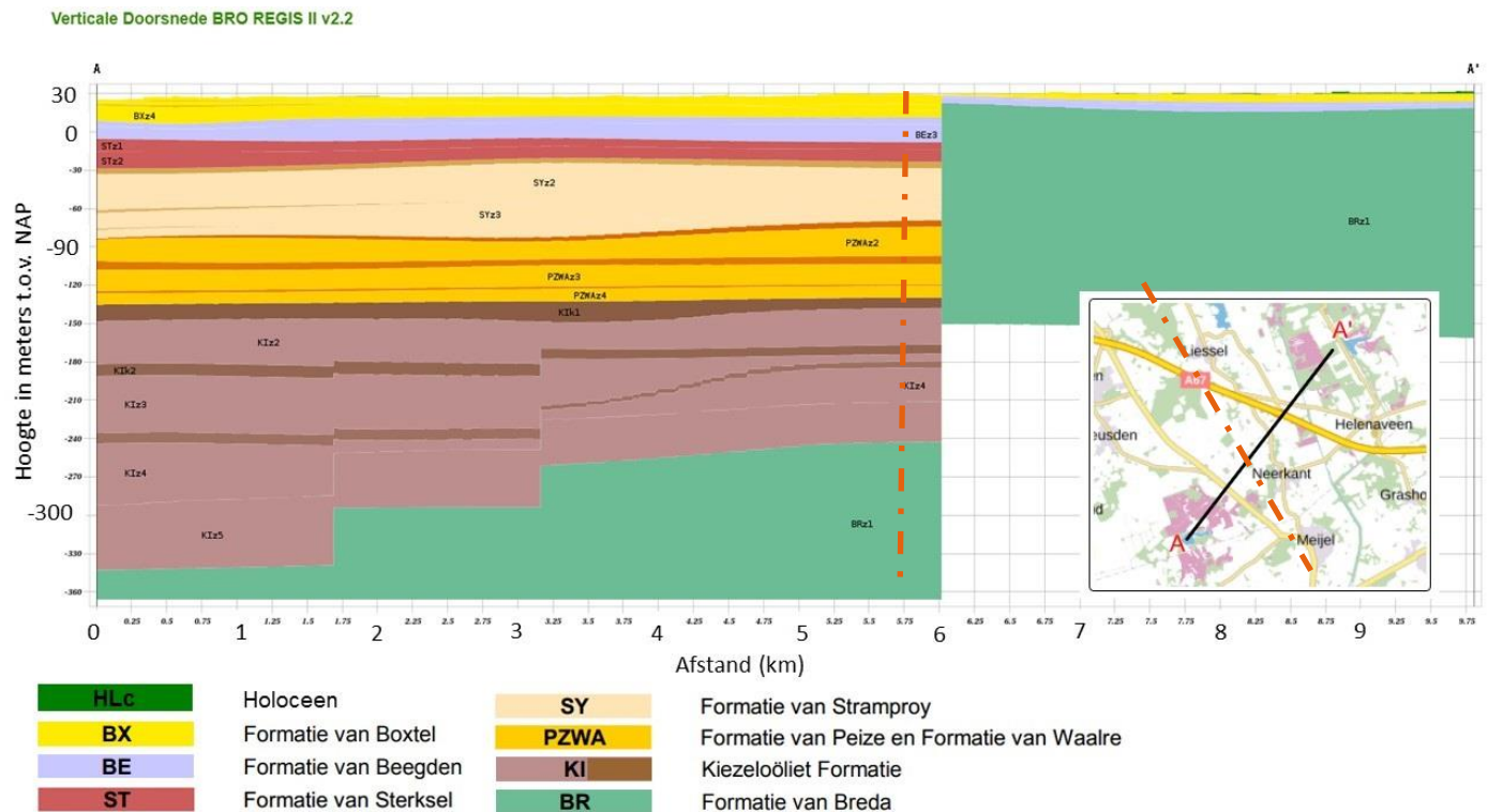
Figuur 3-8 Dwarsdoorsnede van de geologische ondergrond in de wijde omgeving van de Groote Peel (Bron: DINO-loket). De Groote Peel ligt in de Centrale Slenk binnen de linkerhelft van de doorsnede. De Peelrandbreuk ligt ter hoogte van km 6. De geohydrologische basis is aangegeven met de groene kleur
