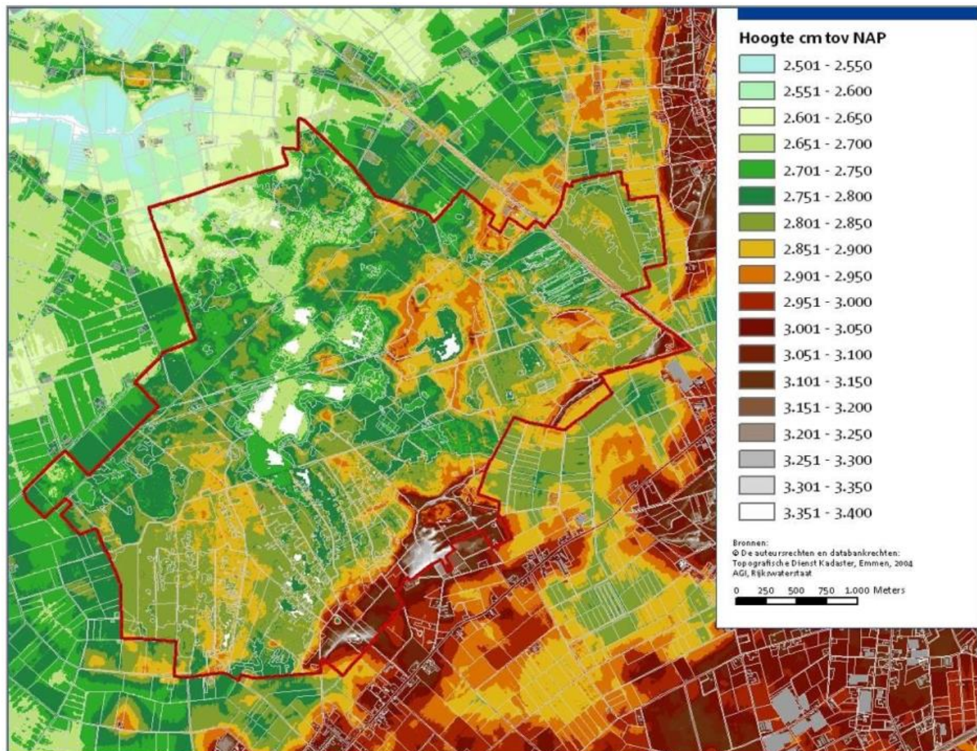
Figuur 3-9 Hoogtekaart van de Groote Peel en omgeving (Bron: DLG & Staatsbosbeheer, 2017)
