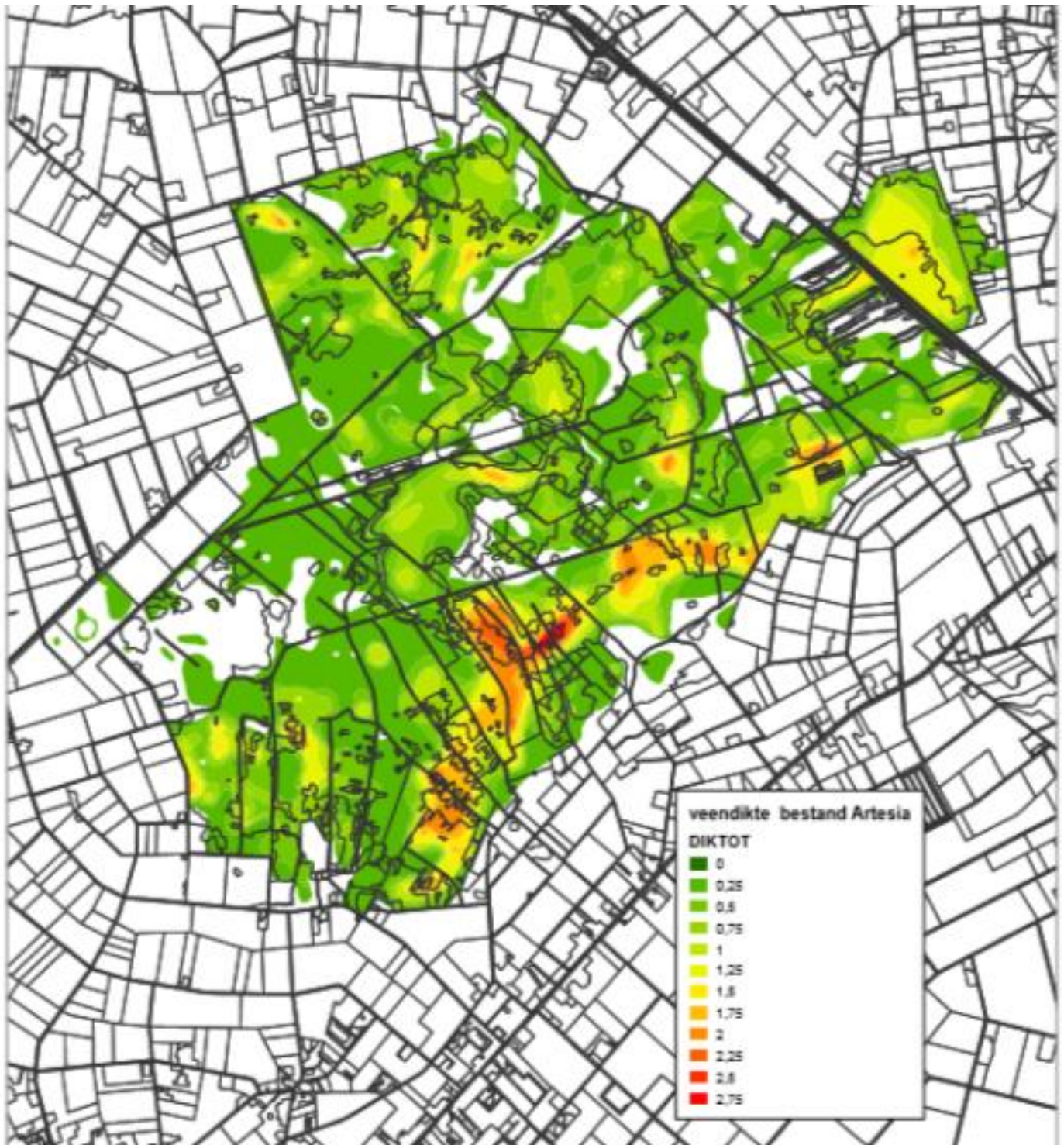
Figuur 3-12 Resterende veendikte in de Grootte Peel, zoals die in 1987 is vastgesteld door Joosten & Lubbers (1988), met interpolatie door Caljé & Beekman (2015)
