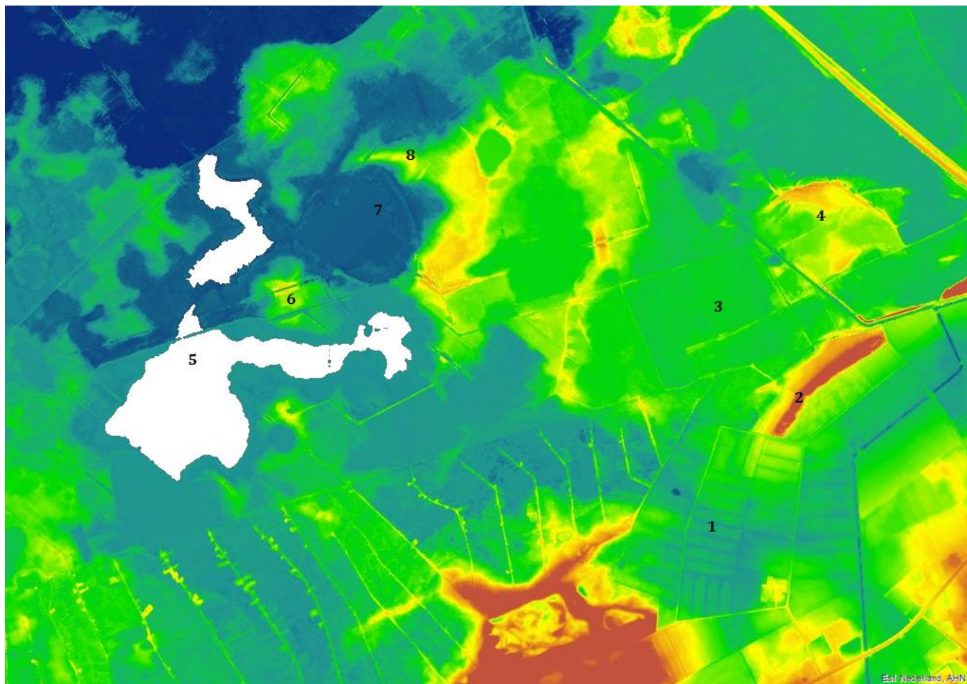
Figuur 3-10 Reliëf in de Groote Peel. Met cijfers zijn de verschillende bij elkaar horende laagten (wit, blauw of groen) en (noordoostelijk daarvan gelegen) hoogten (geel of bruin) te herkennen. 1 en 2 = Kalispeel en Vossenbergh, 3 en 4 = Eeuwig Leven en Berkenbruin, 5 en 6 = Aan 't Elfde en Koeuierberg, 7 en 8 = Koeuerven en Paraboolduin. Bron: ESRI en AHN, overgenomen uit Van Duinen & Joosten, 2019. Dit is een detail van de Groote Peel, binnen de N2000-begrenzing (die daarom niet is weergegeven). Deze figuur laat de relaties tussen de 'gepaarde' hoogtes en laagtes zien
