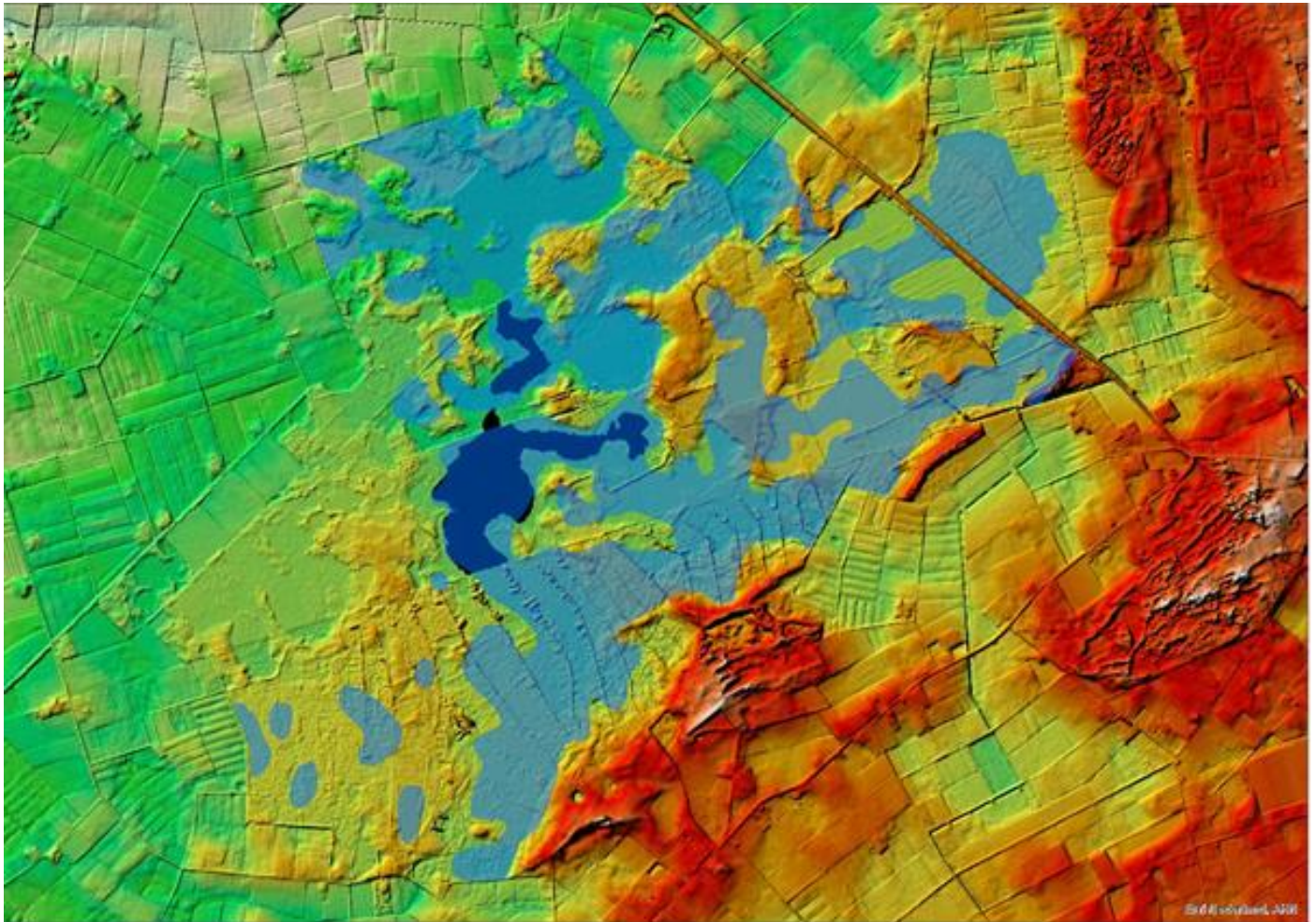
Figuur 3-5 Voorkomen van veen in de Groote Peel dat gevormd is onder invloed van grond- en/of oppervlaktewater (lichtblauw; Bron: Joosten & Bakker, 1987) met een hoogtemodel (Bron: ESRI en AHN) als ondergrond. Rood en geel, hoge gronden; groen en grijs, lage gronden. Donkerblauw zijn de huidige grote open wateren 't Elfde en Steltlopersven. Overgenomen uit: Van Duinen & Joosten, 2019
