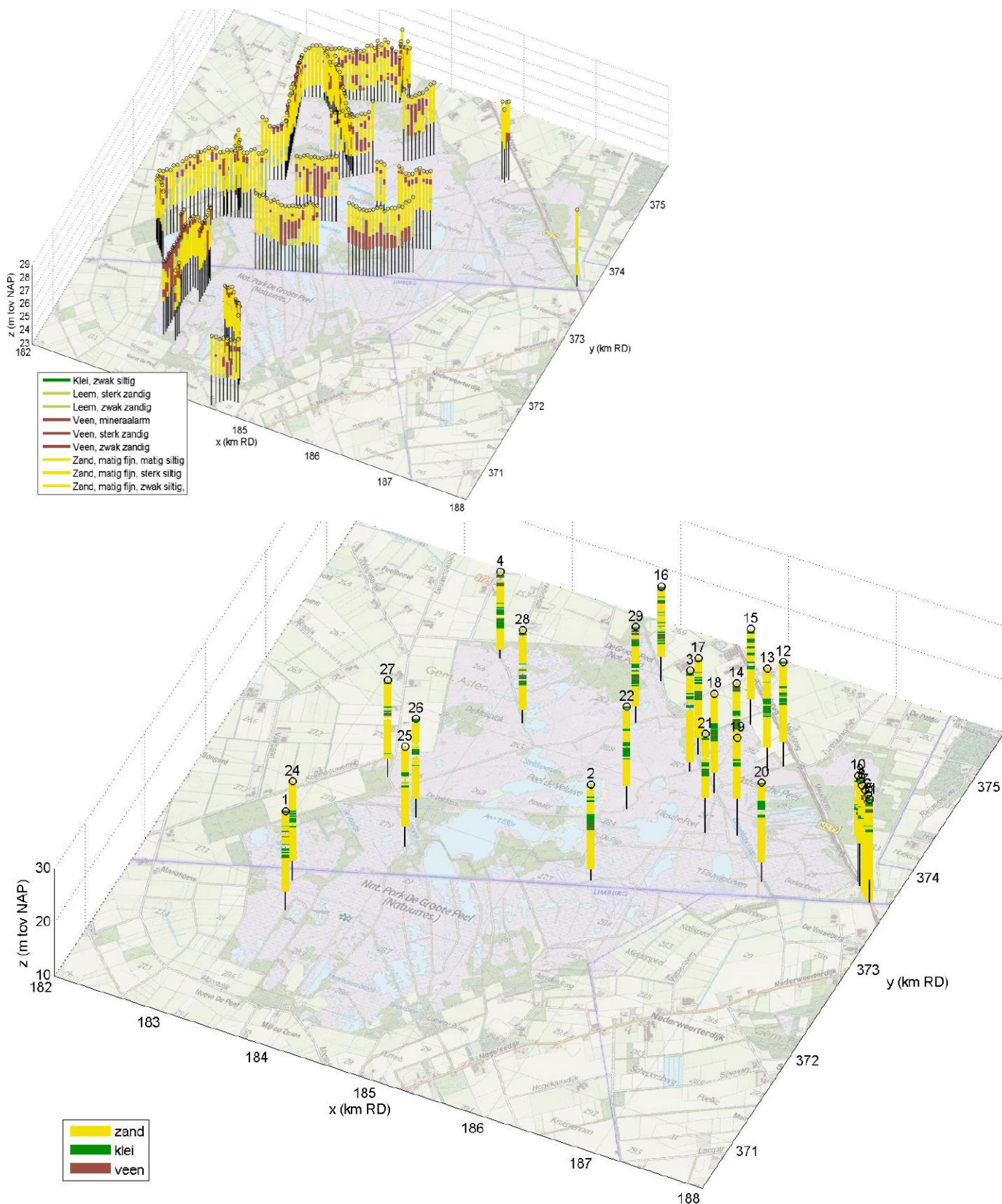
Figuur 3-7 De in bodemboringen waargenomen veenlagen (bruin) en klei- en leemlagen in de Groote Peel (donker en licht groen in de afbeeldingen). Bron: Caljé, 2016
