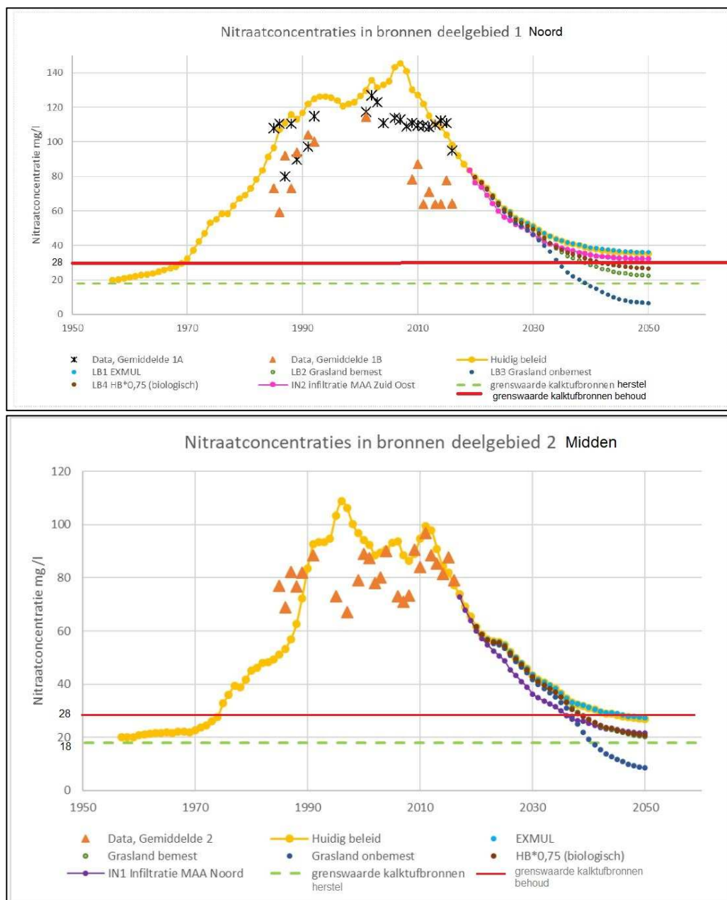
Figuur 7 Verloop gemiddelde nitraatconcentraties in de kalktufbronnen voor deelgebied Noord (boven) en Midden (beneden) bij verschillende scenario's op basis van een regionaal model (van de Weerd 2018).
