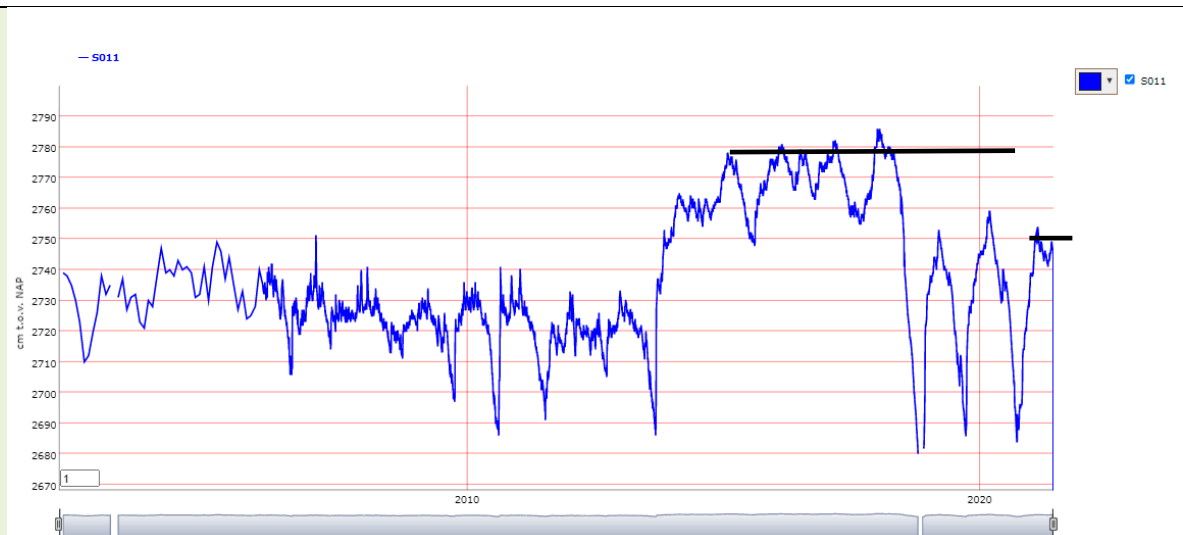
Figuur 2: Oppervlaktewaterpeil in het hoogveencompartiment van het Vragenderveen S011 naast schotbalkstuw (bron: Waterweb)
