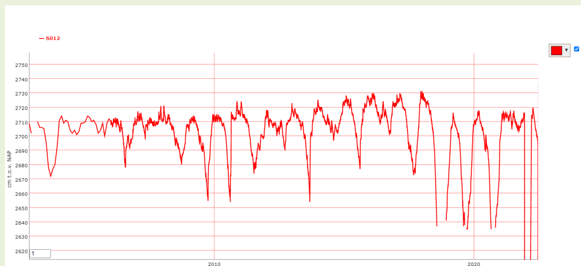
Figuur 3: Peilverloop S012 (stuw ten westen van Galigaanmoeras)
