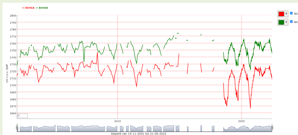
Figuur 2: Peilverloop in het Vragenderveen bij meetpunt B046A (filter in zandlaag onder het veen) en B046B (ondiepe filter in het veen); bron: Waterweb
